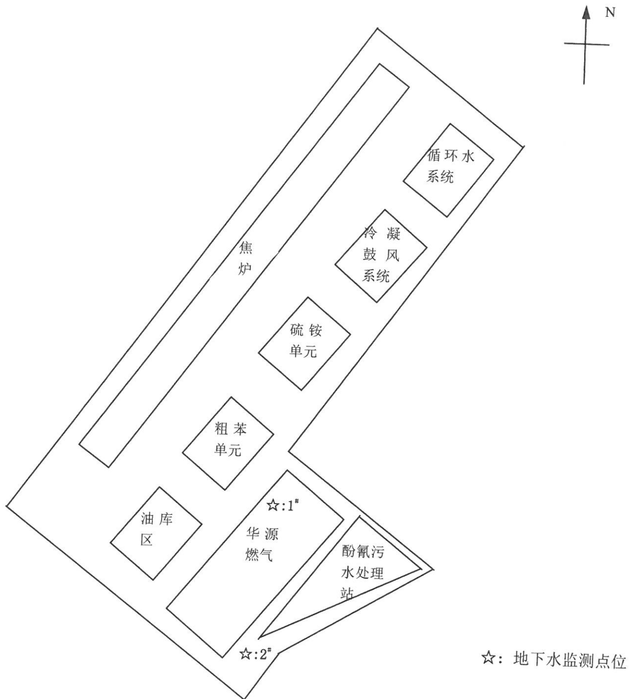
图 4-1 地下水监测点位平面示意图
